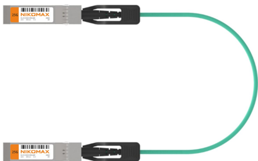
АОС кабель NIKOMAX SFP28, 25 Гбит/с, 850 нм, 3 м
