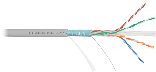
Кабель NIKOMAX F/UTP, 4 пары, Кат.6а, 23 AWG, внутренний, поливинилхлорид, 500м
