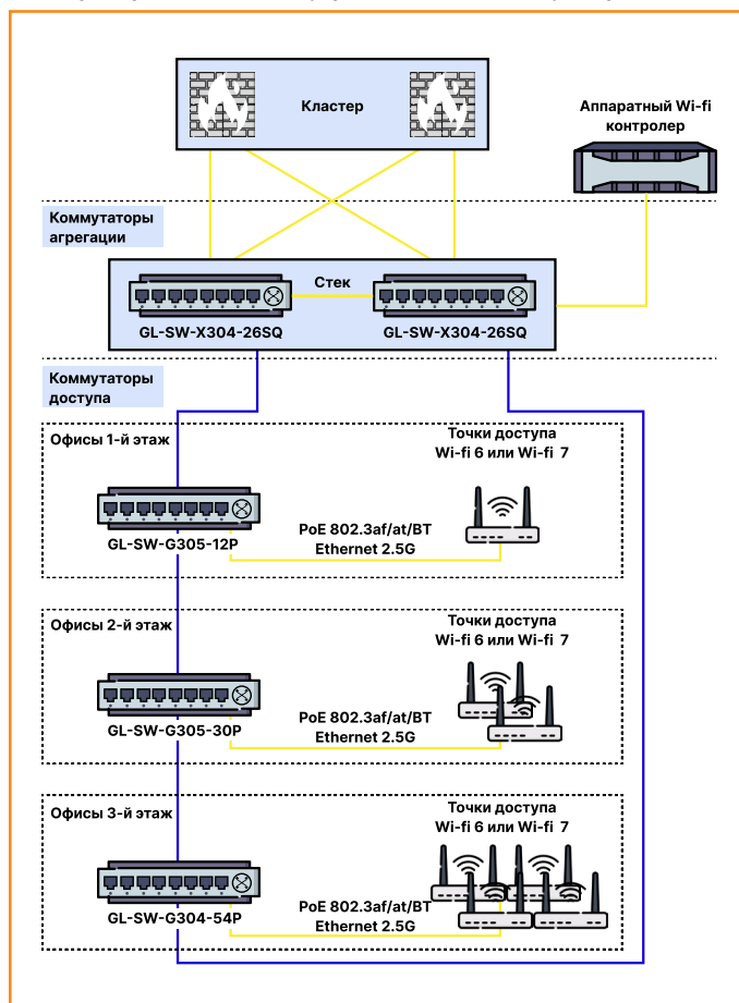
Пример использования управляемых PoE коммутаторов 2.5G
