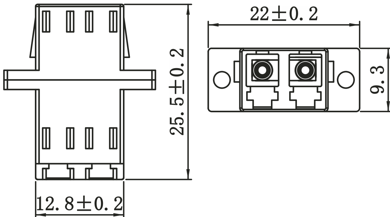
Габаритный чертеж
