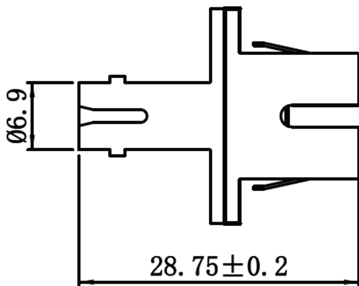
Габаритный чертеж
