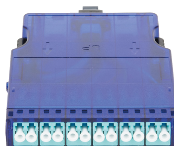
NMF-CJ12M3PA-MTPM-LCU-1S 1 слот, MM 50/125 OM3, 1x MTP / male - 12x LC / UPC, полярность A
