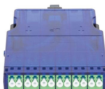
NMF-CJ12S2PA-MTPM-LCA-1S 1 слот, SM 9/125 OS2, 1x MTP / male - 12x LC / APC, полярность A
