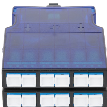
NMF-CJ12S2PA-MTPM-SCU-2S 2 слота, SM 9/125 OS2, 1x MTP / male - 12x SC / UPC, полярность A
