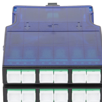
NMF-CJ12S2PA-MTPM-SCA-2S 2 слота, SM 9/125 OS2, 1x MTP / male - 12x SC / APC, полярность A
