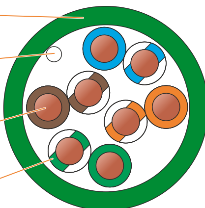
U/UTP
