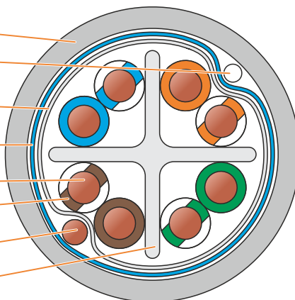
F/UTP
